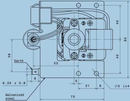
CP08 PACK ALARM TEKNİK ÇİZİMİ
