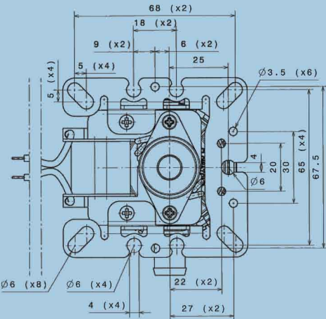
CP08SC6641 TEKNİK ÇİZİMİ
