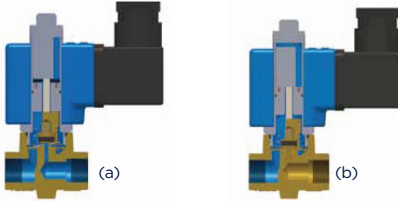
Şekil 10: Normalde açık vananın çalışması, (a) enerji yokken, (b) bobinde enerji varken.
