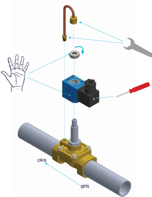
Şekil 14. Borulu tip solenoid vana montajı
